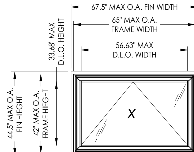
FIN MOUNT
